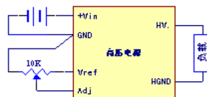
电位器调节
